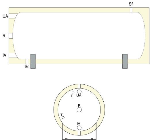
BOLLITORE INOX ORIZZONTALE SENZA FLANGIA H INX OS
