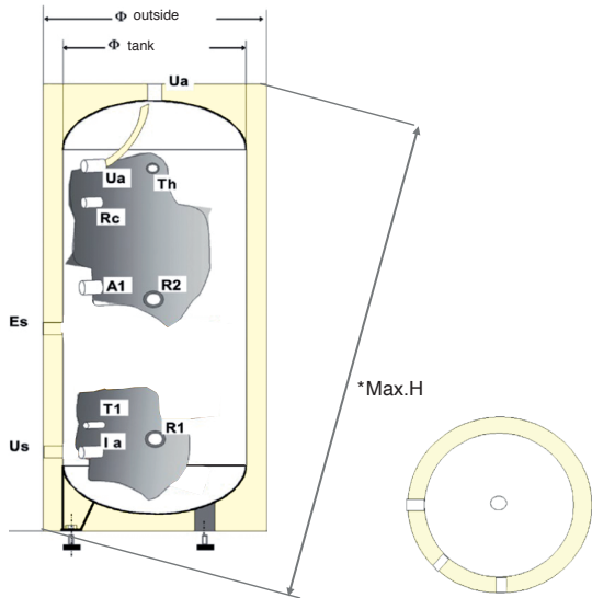
BOLLITORE INOX VERTICALE SENZA FLANGIA INX OS
