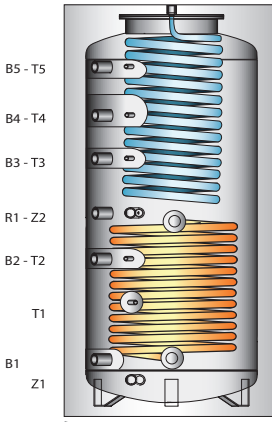
PUFFER CON SCAMBIATORE SANITARIO + 1 SERPENTINO FISSO PESAN 1S
