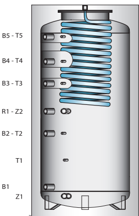
PUFFER CON SCAMBIATORE SANITARIO ESTRAIBILE PESAN OS
