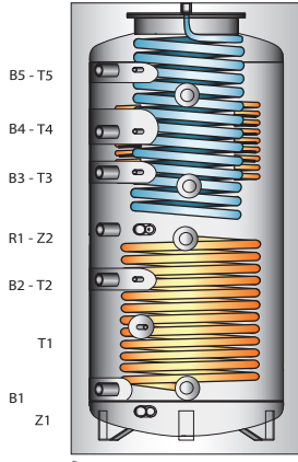
PUFFER CON SCAMBIATORE SANITARIO + 2 SERPENTINI FISSI PESAN 2S
