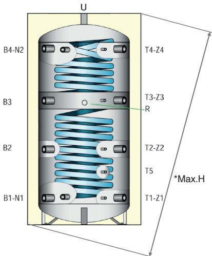
PUFFER CON SERPENTINO SANITARIO POTENZIATO P SAN P OS
