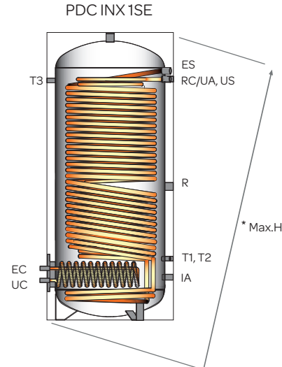
BOLLITORE INOX CON SERPENTINO FISSO MAGGIORATO + SCAMBIATORE SOLARE ESTRAIBILE
