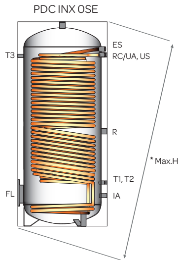
BOLLITORE INOX CON SERPENTINO FISSO MAGGIORATO
